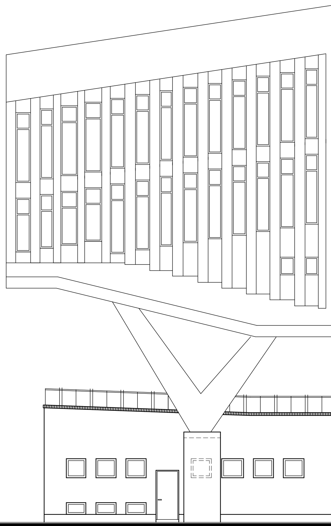
ELEWACJA SALI BŁĘKITNEJ OD UL. LUBOMELSKIEJ 1:100
