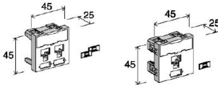
Przykład płyty czołowej (ramki montażowej) 2xRJ45 oraz 1xRJ45
