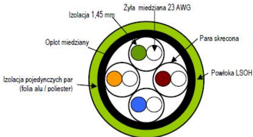
Konstrukcja (przekrój) kabla S/FTP (PiMF) kat. 7 LSOH
